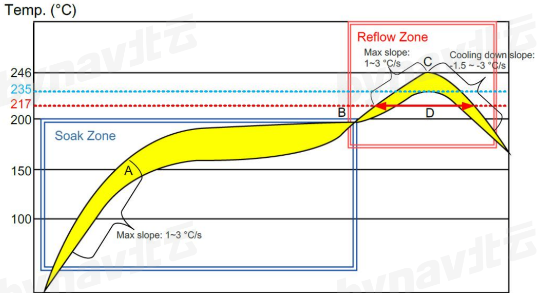
图 8- 2 装配推荐炉温曲线
