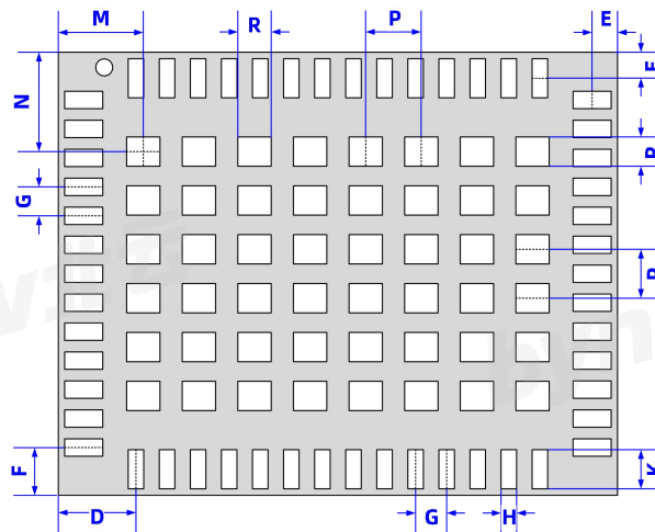
图 9- 1 模组外形图
