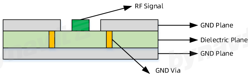
图 6- 1 Coplanar waveguide 平面传输线结构示意图
