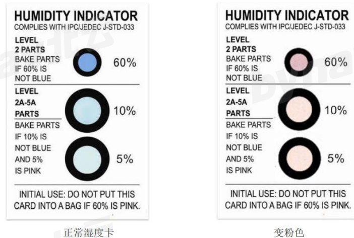
图 8- 1 三点湿度指示卡
