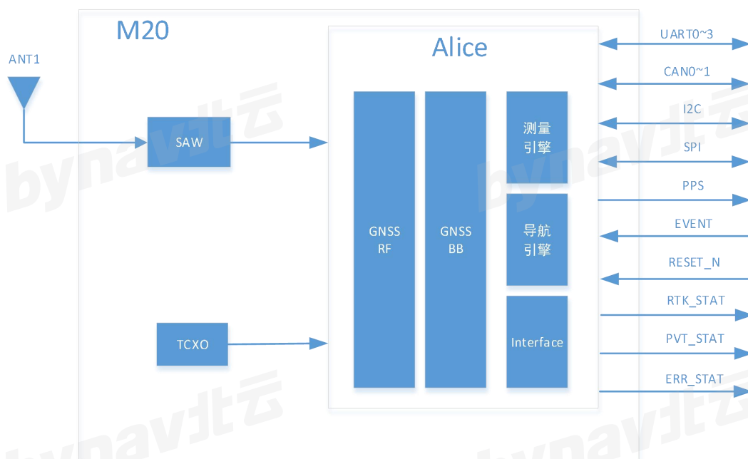
图 2- 1 架构框图
