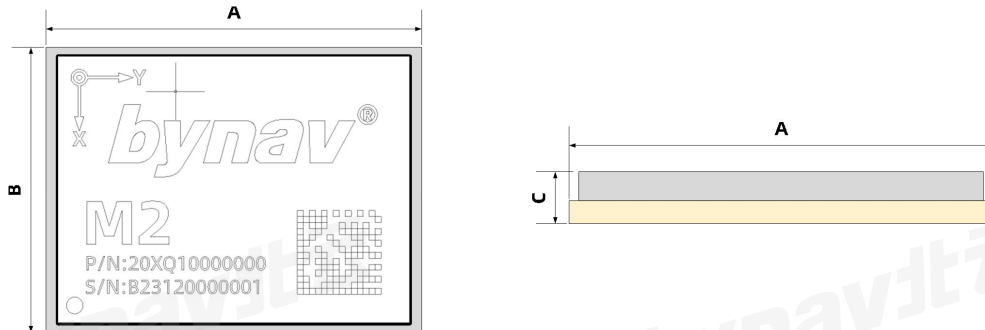
图 9- 1 模组外形图
