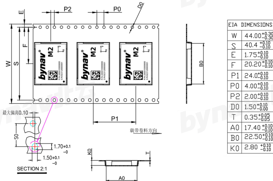
图 11- 1 载带信息
