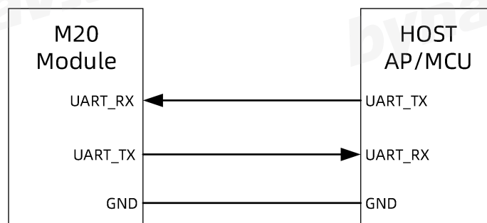
图 6- 11 推荐 UART 设计
