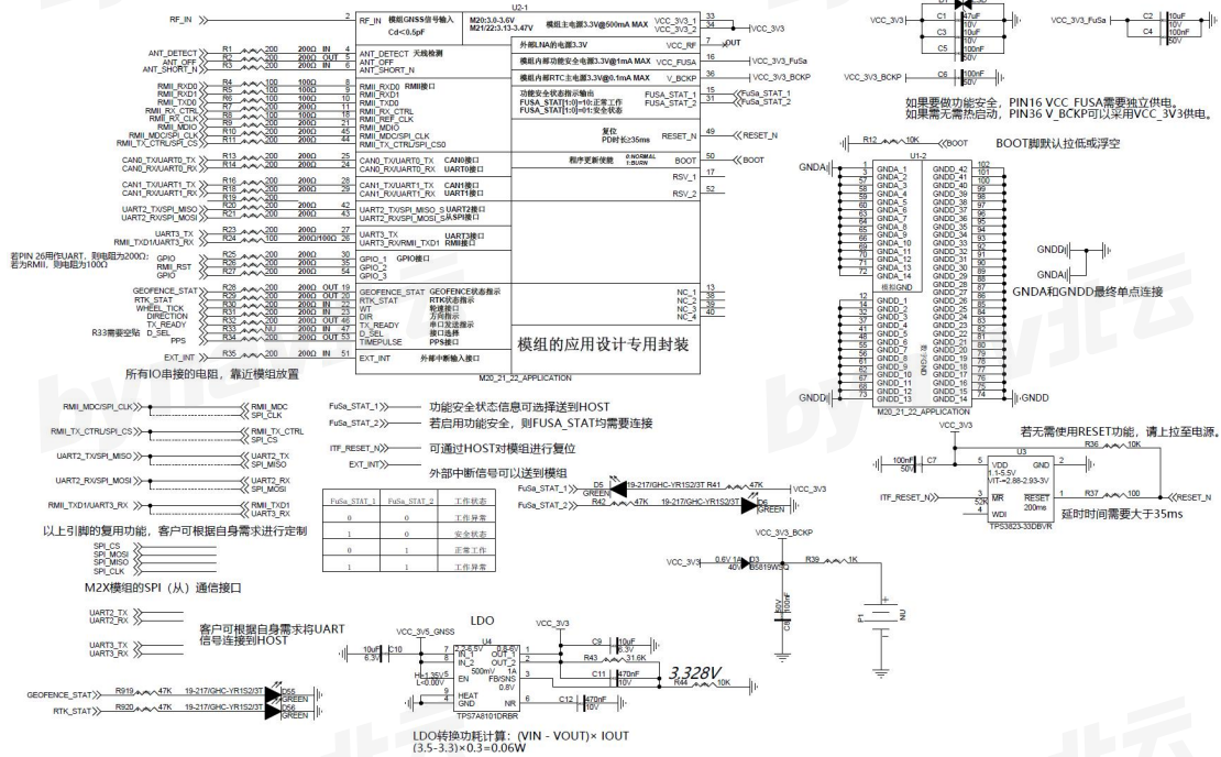
图 13- 1 M20 部分参考设计
