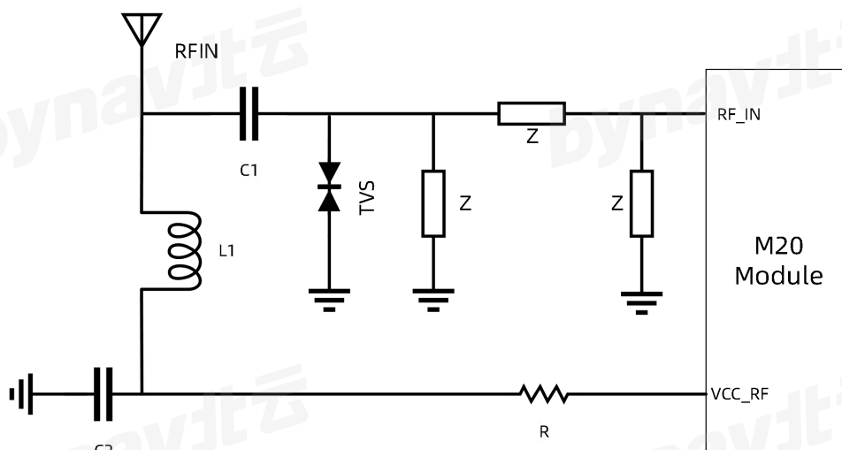
图 6- 6 有源天线的参考设计
