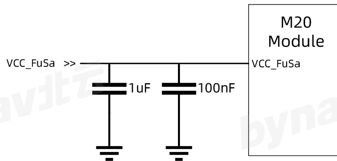
图 6- 9 推荐 FuSa 电源设计
