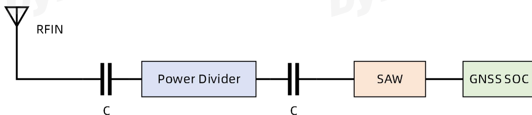
图 6- 2 内部射频前端结构
