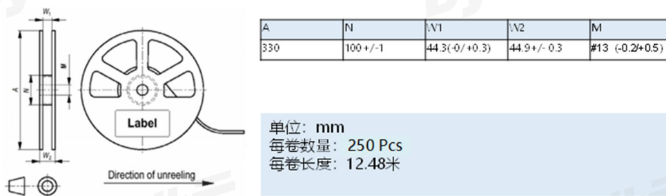
图 11- 2 卷盘信息
