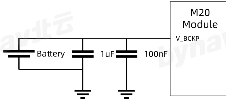
图 6- 8 推荐 V_BCKP 设计
