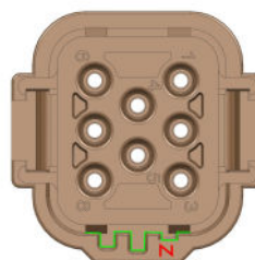
Z-Keying*
