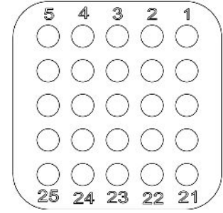
25 Way=25*#16
