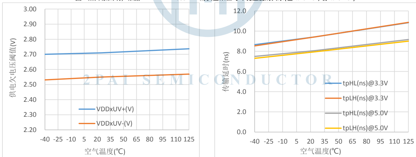
图 8.UVLO vs. 空气温度
