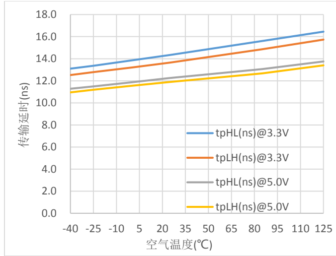
图 10.π16x6x 传输延时 vs. 空气温度
