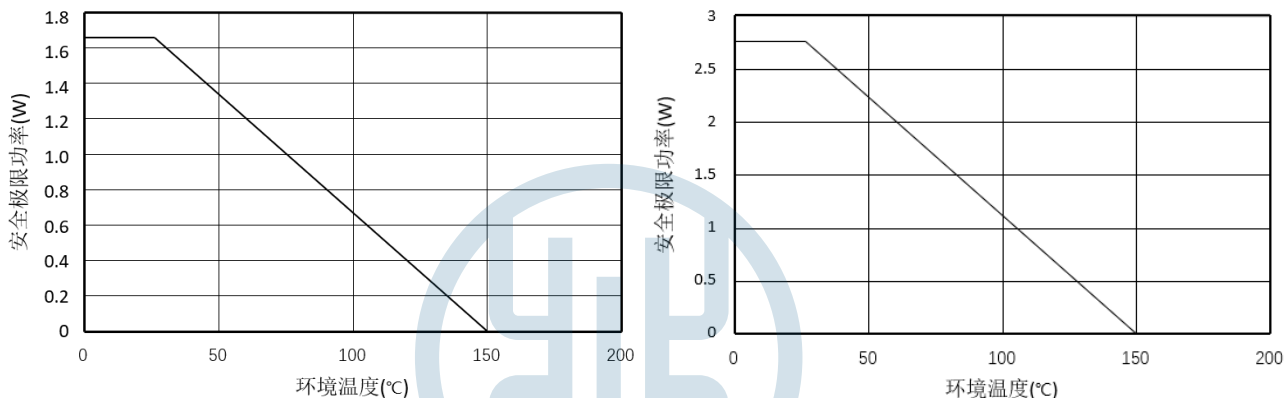
图 7.热降额曲线, 依据 DIN V VDE V 0884-11 的安全限值与环境温度的关系(左: π16xE3x; 右: π16xE6x)
