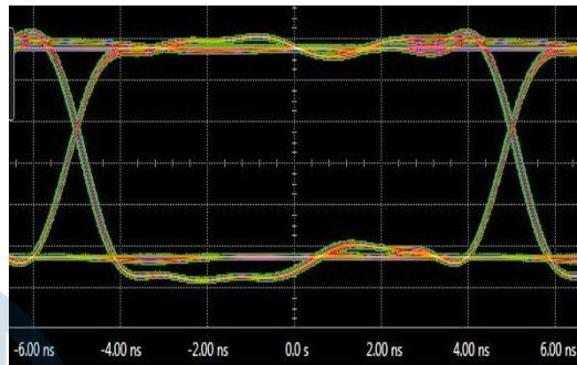
图 14. \pi 16XEXX 眼图
