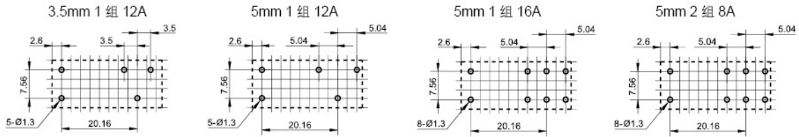
安装孔尺寸 PCB Layout( 底视 Bottom View)
