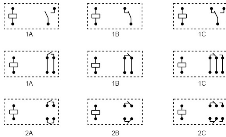
接线图 Wiring Diagram( 底视 Bottom View)
