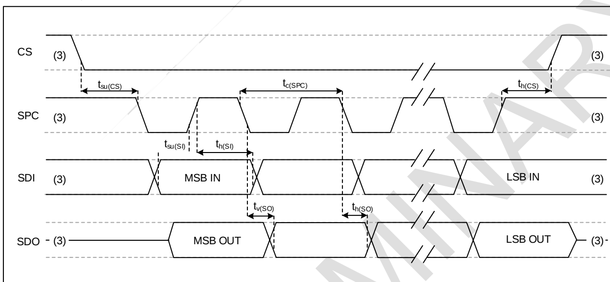
SPI 从设备时序图
