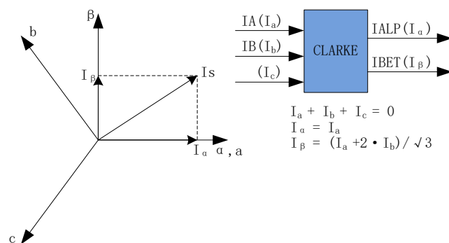
图 12-4 CLARKE 变换
