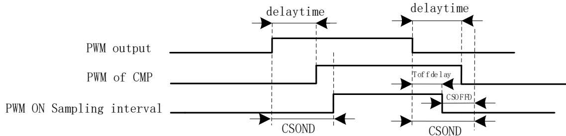
图 27-14 PWM ON 采样模式
