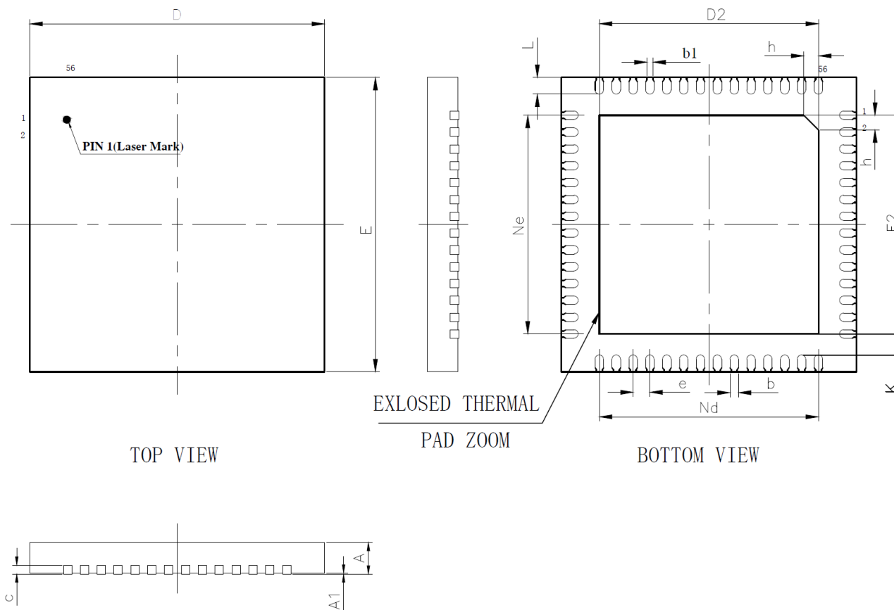
图 34-2 QFN56_7X7 封装尺寸图
