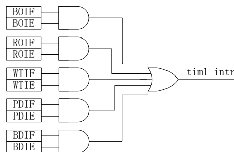
图 14-12 TIMER1 中断源
