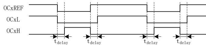
图 18-5 带死区插入的互补输出
