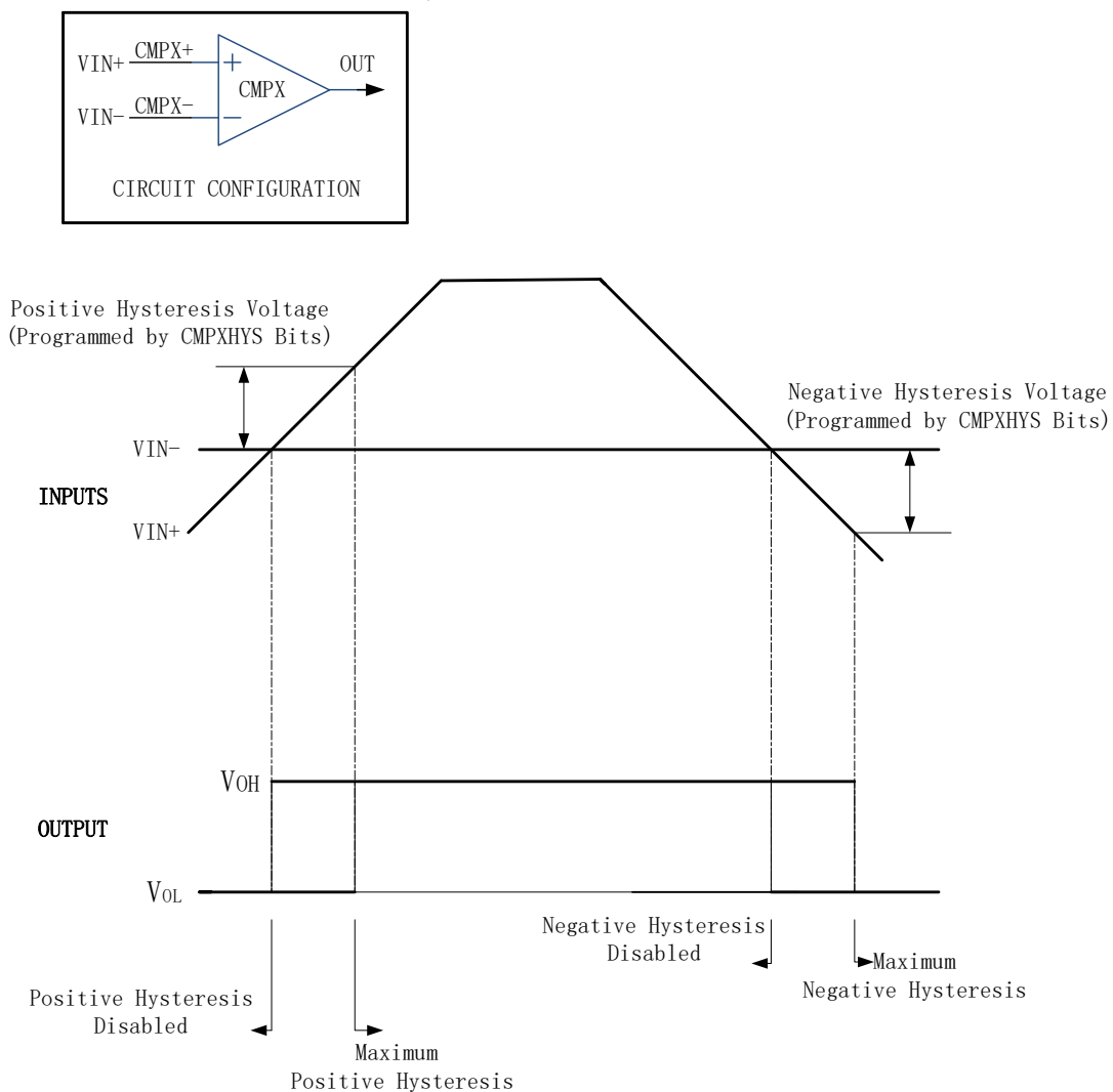
图 27-13 比较器 0 迟滞输入输出图
