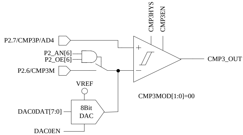
图 27-2 CMP3MOD[1:0]=00B, 选择单比较器输入模式
