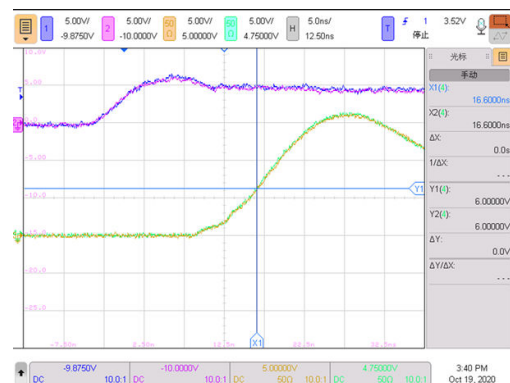
Figure 20. Rising Edge
