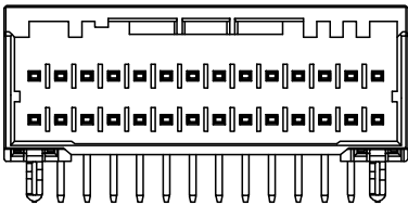
28POS: 560UBG-001H****T000
