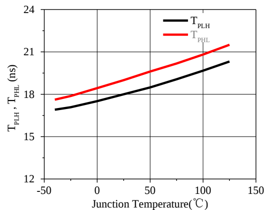
(f) T_{PLH} , T_{PHL} VS T_J
