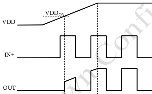
图2 上电过程
