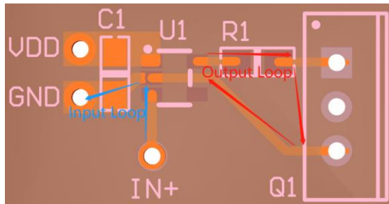
图 3 布局举例
